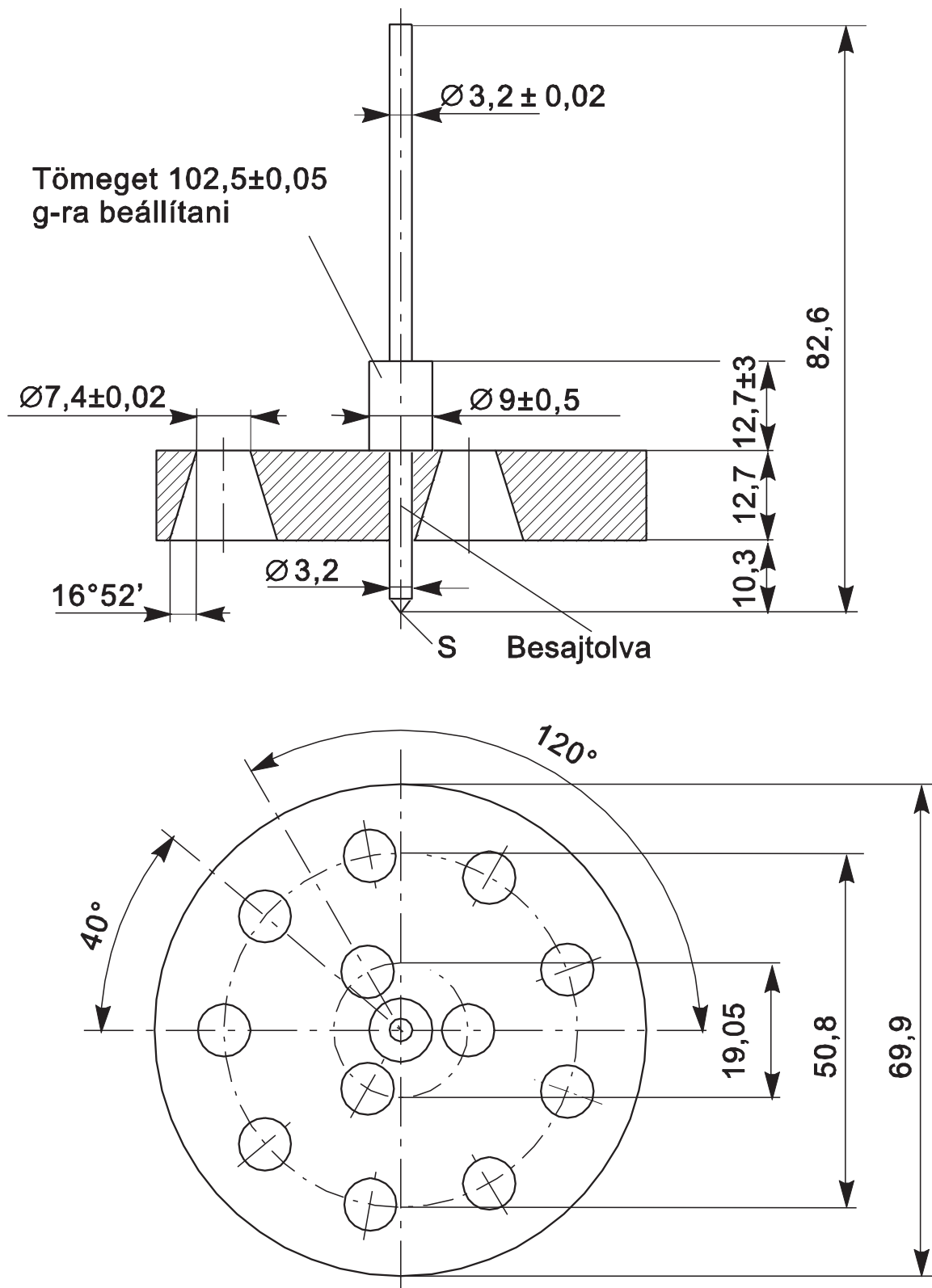
4. ábra: Penetrométer
