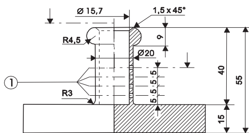
3. ábra: Talpas bronzhenger, egyik végén zárt: felülnézet és oldalnézet metszettel, méretek mm-ben
