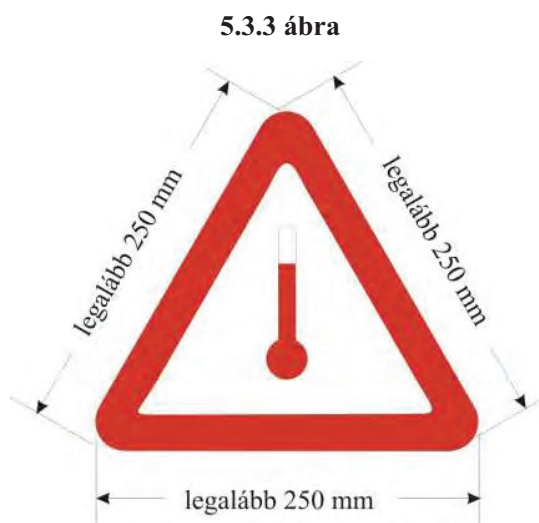
Magas hőmérsékleten szállított anyag jelölése
