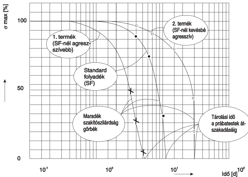
3. ábra Feszültségi repedés vizsgálat (csapbenyomásos módszer)
